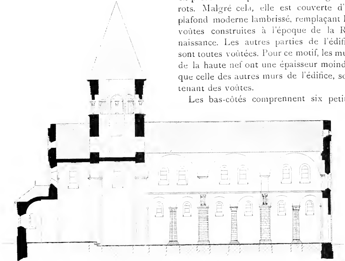
Eglise de Saint-Séverin. Coupe longitudinale (d'après M. L. 1906, p. 10).
